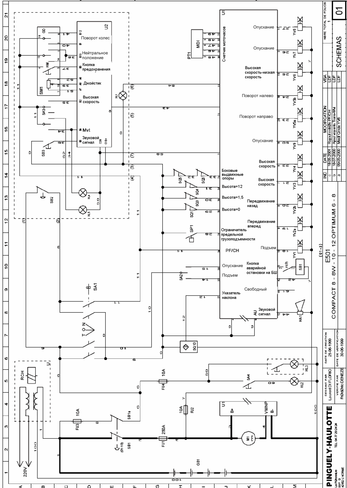
Рисунок 31. Электрическая схема подъемника Compact 8.
