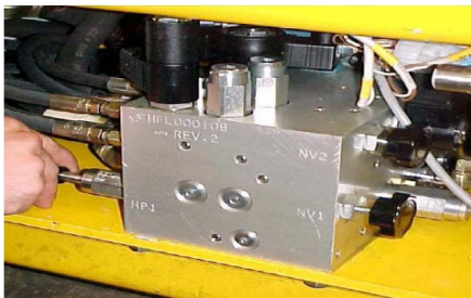
Рисунок 24. Аварийное растормаживание колес подъемника.
